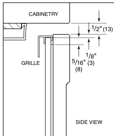
Grille Top
